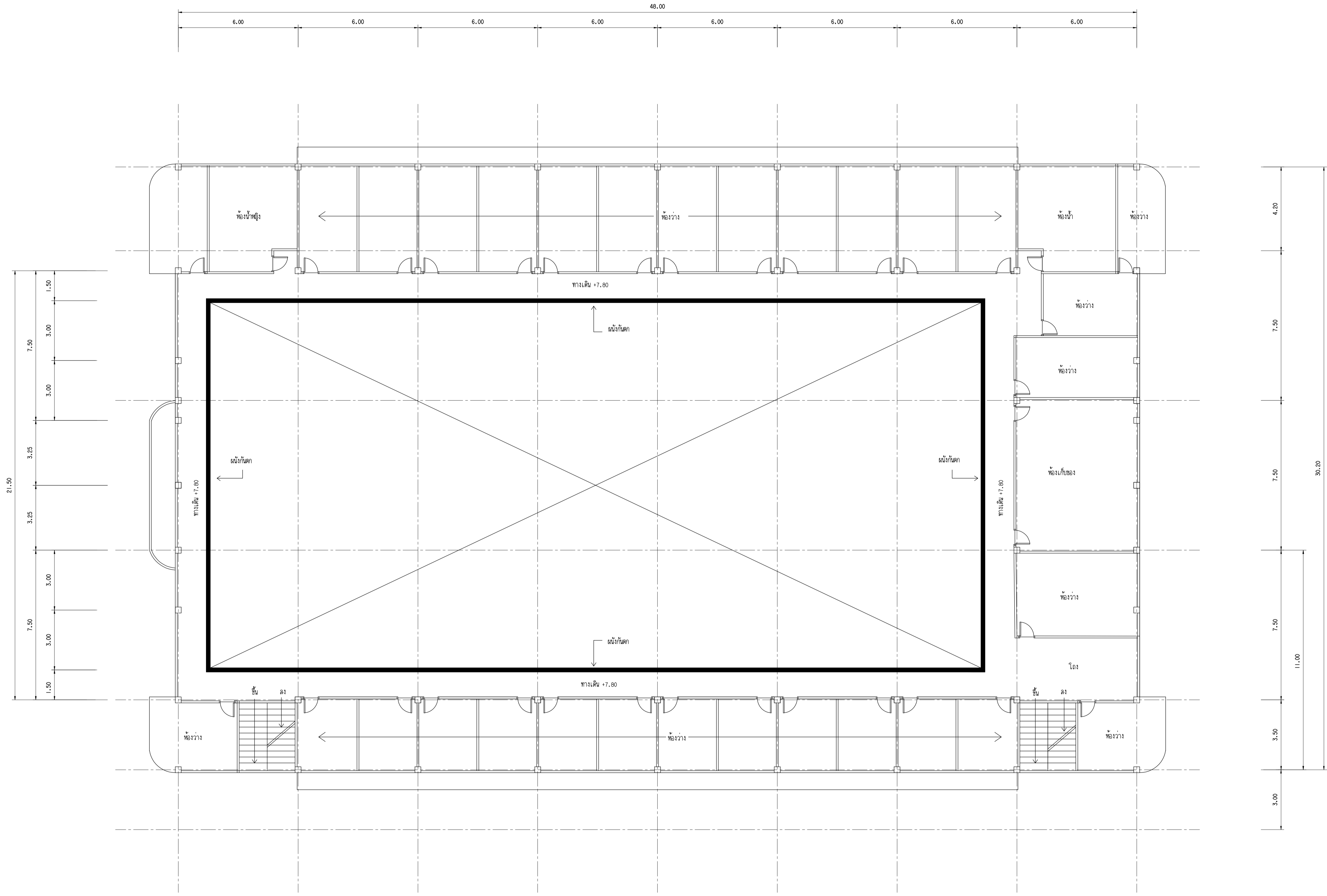
แปลนพื้นที่ 3 อาคาร 37 เทคนิคกรุงเทพฯ มาตรฐาน 1 : 100 ก่อนปรับปรุง
