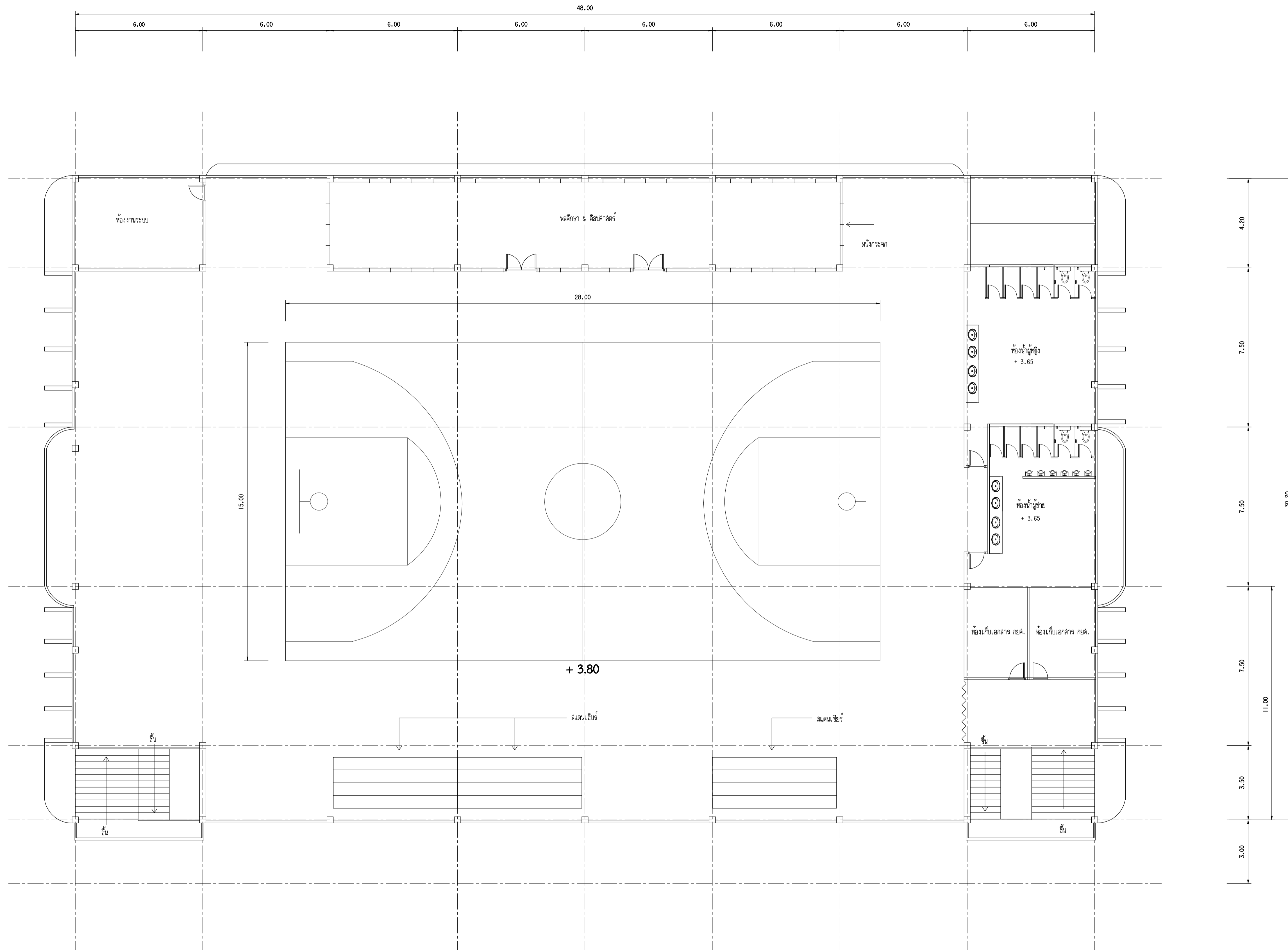
แปลนพื้นที่ 2 อาคาร 37 เทคนิครุงเทพฯ มาตรฐาน 1 : 100 ก่อนปรับปรุง
