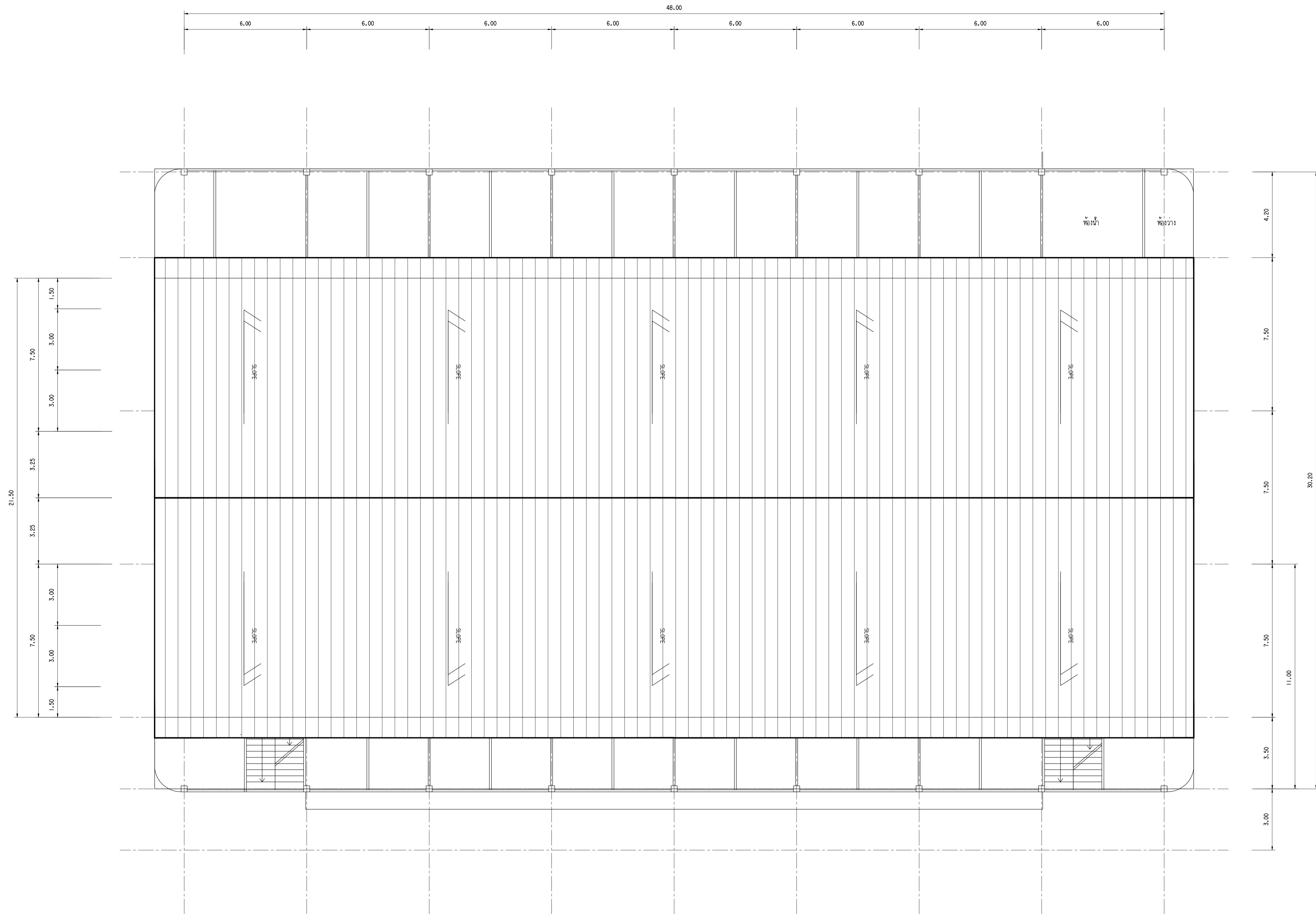
แปลนพื้นที่ ดาดฟ้า อาคาร 37 เขตคันจิ กรุงเทพฯ มาตรฐาน 1 : 100 ก่อนปรับปรุง
